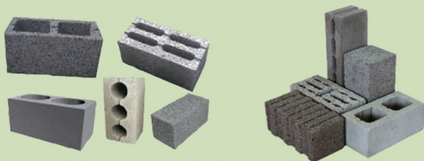
керамзитобетонные блоки
